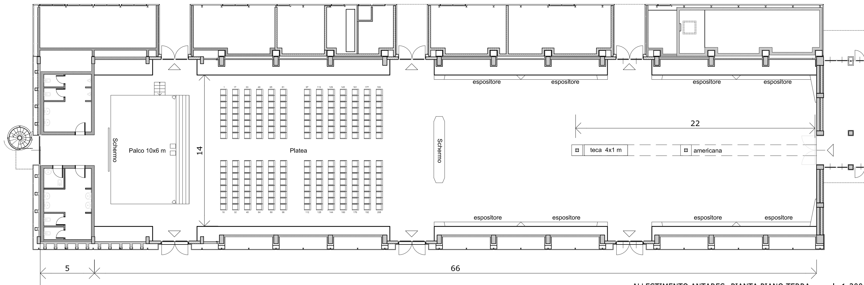
ALLESTIMENTO ANTARES; PIANTA PIANO TERRA - scala 1:200
