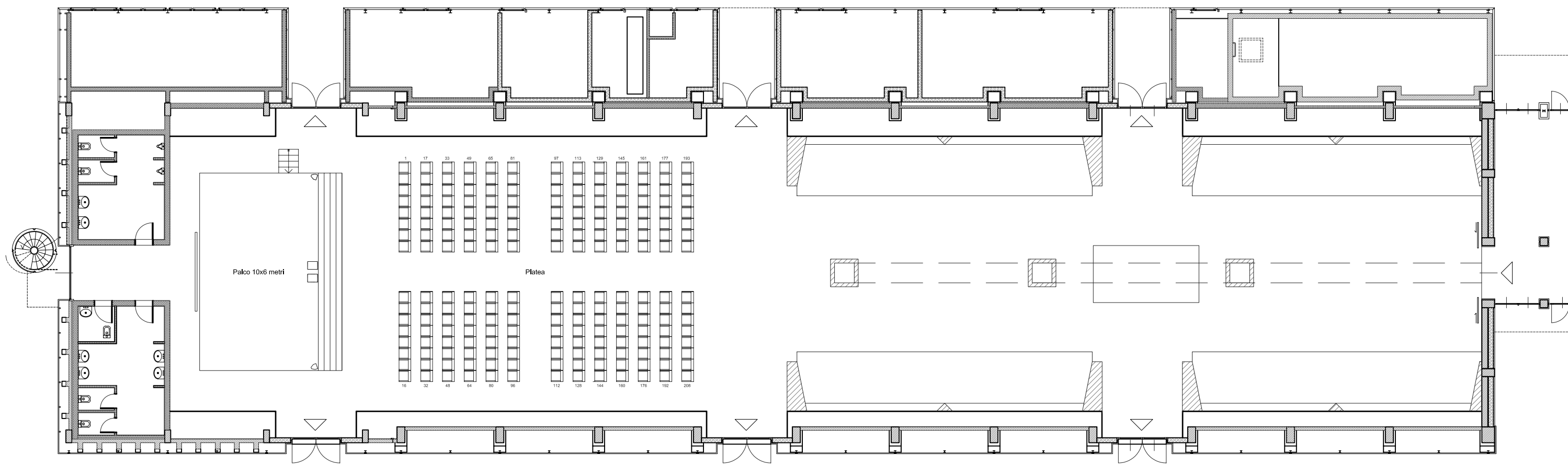
ALLESTIMENTO ANTARES; PIANTA PIANO TERRA - scala 1:200
